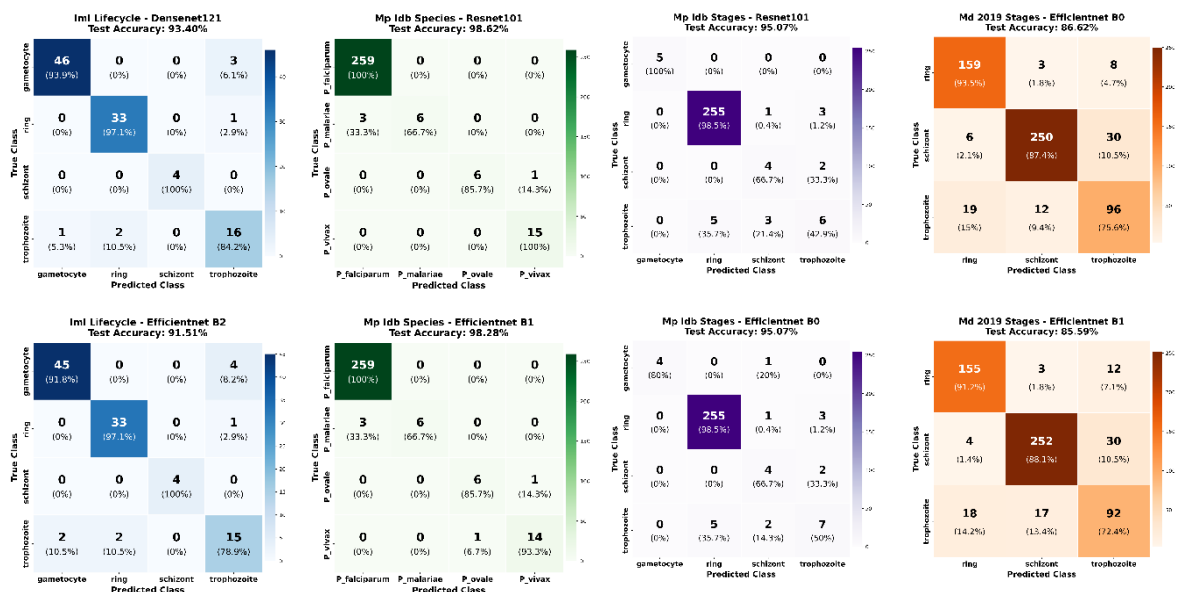
Gambar 4 Confusion Matrices - Performa Klasifikasi pada 4 Dataset
